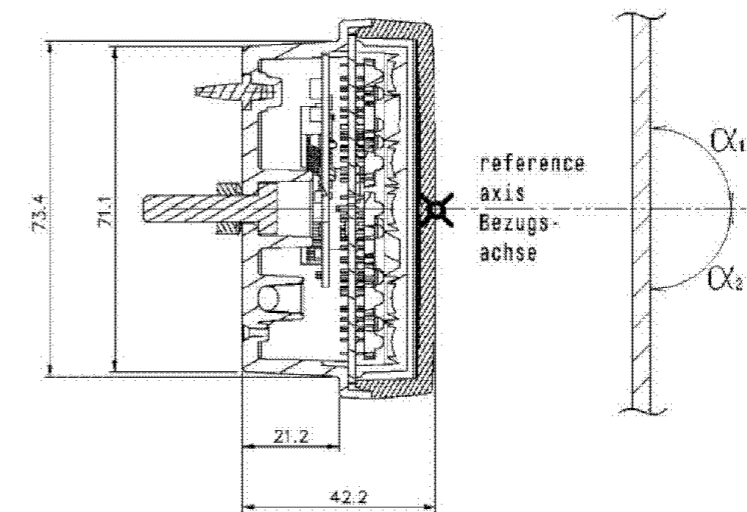
Top - View Ansicht von oben
